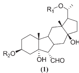
R 1 : β-D-glucopyranose
