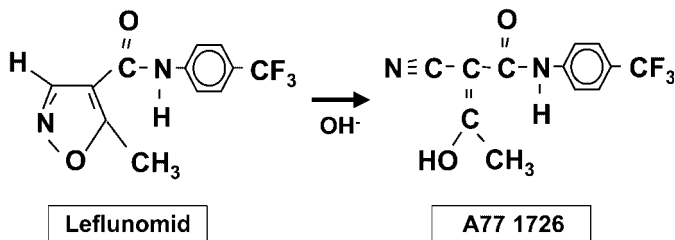
Abb. 1 Chemische Strukturformeln für Leflunomid (Molekulargewicht 270 Da) sowie dessen aktiven Metaboliten A77 1726.
