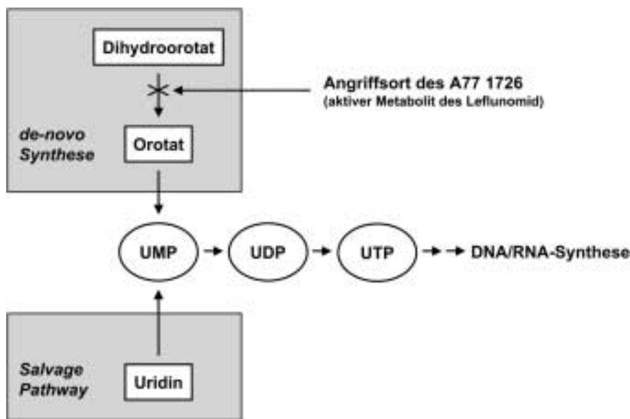
Abb. 2 Einfluss des Leflunomid-Metaboliten A77 1726 auf die Nucleinsäure-Synthese über die direkte Hemmung des Enzyms Dihydroorotatdehydrogenase. Dieses Schlüsselenzym der De-novo-Synthese der Pyrimidine katalysiert den Umbau von Dihydroorotat zu Orotat, der Grundsubstanz zum Aufbau von Uridinmonophosphat (UMP). UMP kann in begrenzter Menge auch durch Verwendung extern zugeführter Uridine synthetisiert werden (Salvage Pathway). Mittels weiterer enzymatischer Reaktionen entsteht aus UMP Uridindiphosphat (UDP) sowie -triphosphat (UTP). UTP ist einer der Grundbausteine der Nucleotidsynthese zum Aufbau von DNA und RNA. Ein Minderangebot an UTP bewirkt somit eine Reduktion der Nucleinsäure-Synthese.
