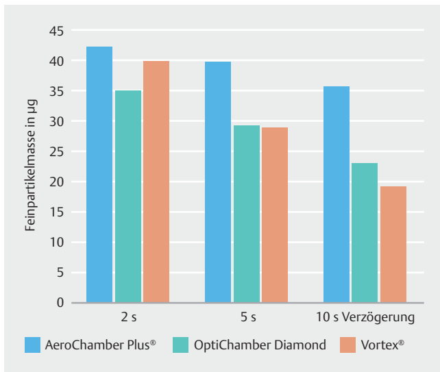
► Abb. 2 Von verschiedenen antistatischen Spacern freigesetzte Feinpartikelmasse. Mittelwerte in µg (FP-HFA, 125 µg) bei verschiedenen Verzögerungszeiten zwischen Dosieraerosolauslösung und Inhalation (nach [36]).
