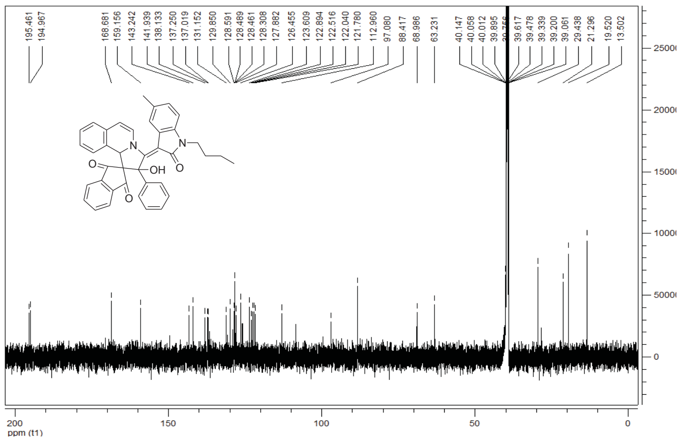
2'-Isatylidene spiro[indan-2,1'-pyrrolo[2,1-a]isoquinoline] 3p
